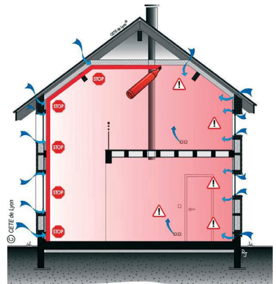
Localisation des fuites d'air récurrentes Source : CETE de Lyon
